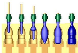
Processus d'étrépage-soufflage d'une préforme. (Extrait de Wikipedia)
